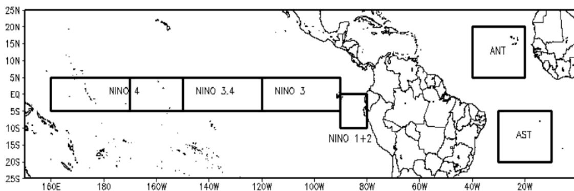
Figura 9 – Regiões de medições de El Niño (EN) e La Niña (LN)
