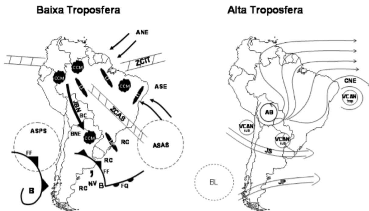
Figura 6 - Representação dos sistemas atmosféricos atuantes na América do Sul
